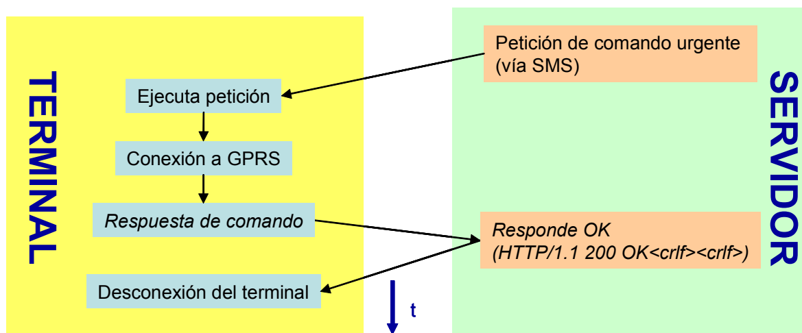
Figura 2 Diagrama de flujo de la atención de peticiones urgentes. Éstas se envían por SMS. En cursiva las acciones que no se llevan a cabo si no se puede establecer conexión GPRS y es una acción no permitida por SMS
