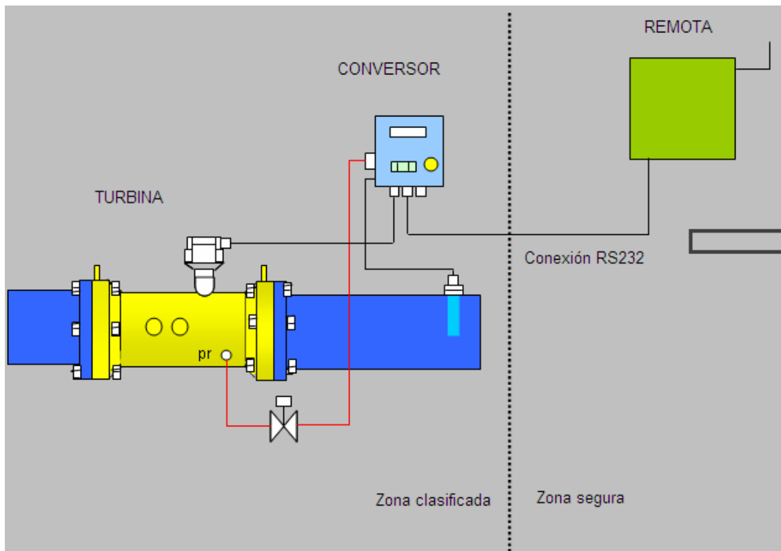
Fig. 4 Conexión remota a convertidor por protocolo.
