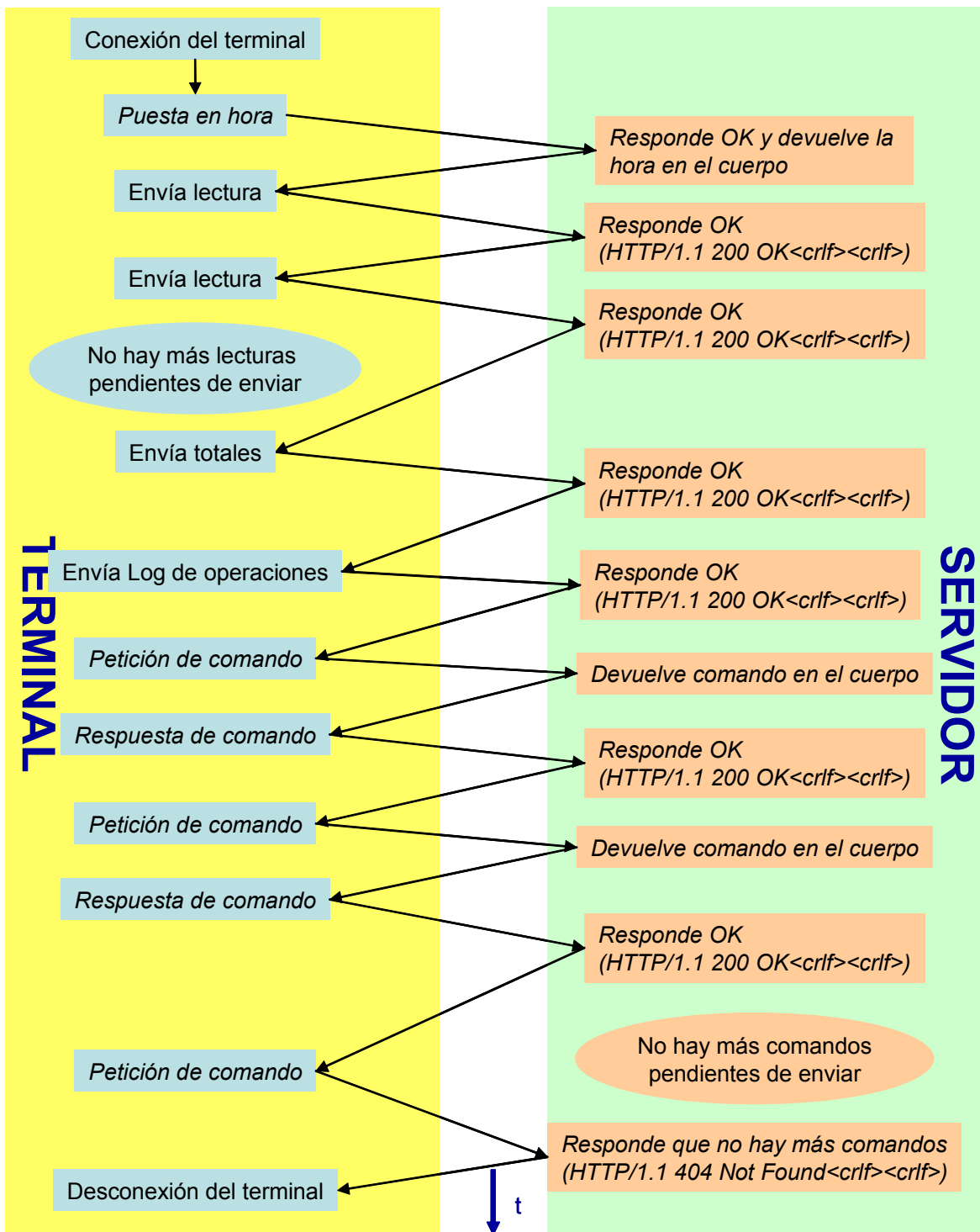
Figura 1 Diagrama de flujo en una conexión estándar vía GPRS. En cursiva las acciones que no se llevan a cabo en caso que no se pueda establecer la conexión GPRS y haya que enviar las lecturas vía SMS.
