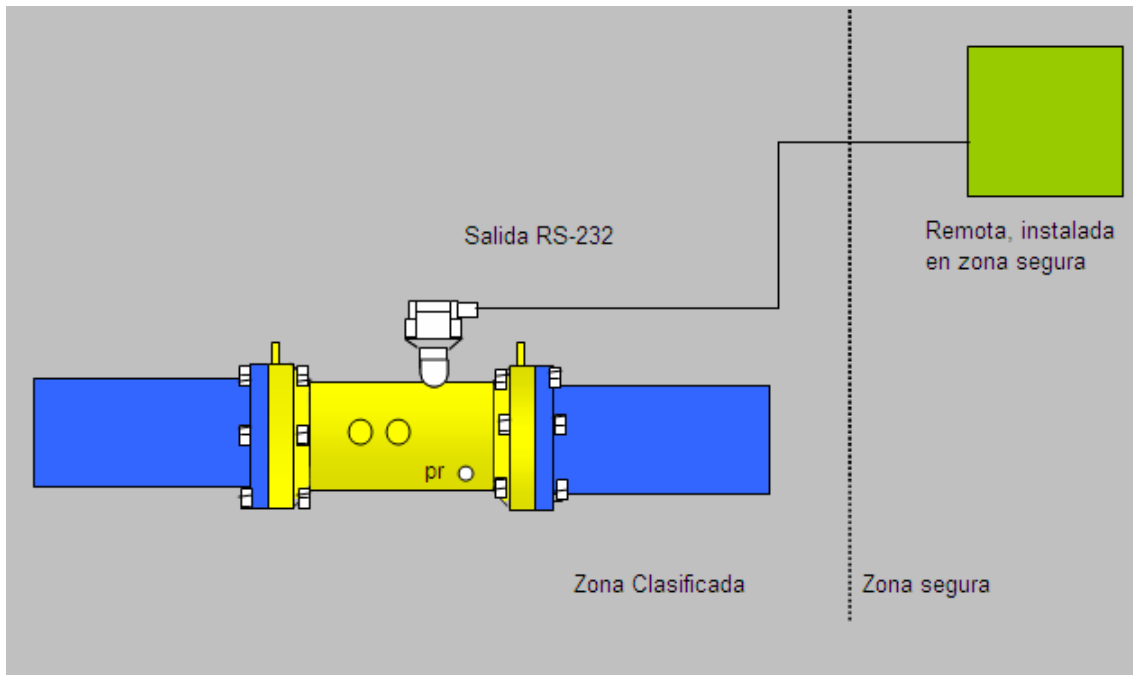
Fig. 3 Medidor de caudal conectada a remota vía RS 232
