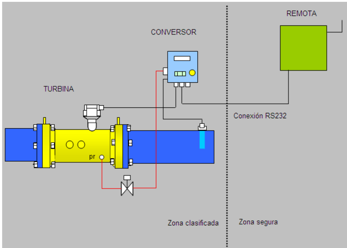
Fig. 1 Remota conectada a convertidor de volumen de gas, instalado en zona clasificada
